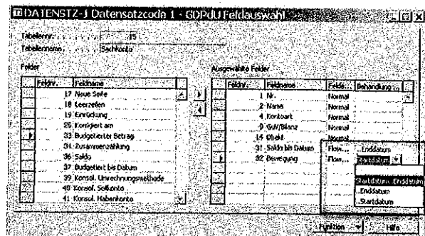
(Abb.2 FlowField definieren)
